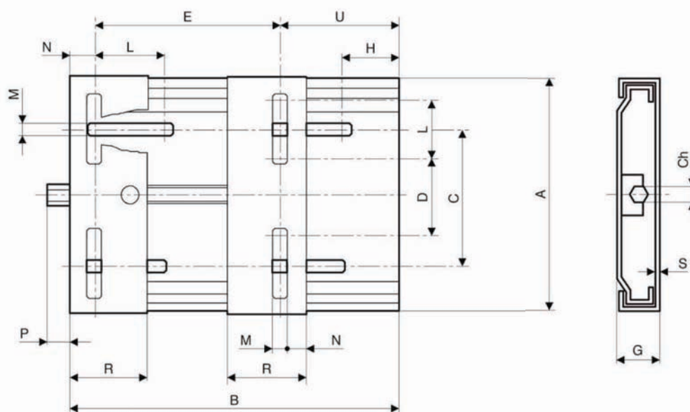
DIMENSIONI / DIMENSIONS / ABMESSUNGEN / DIMENSIONS / DIMENSIONES [mm]
